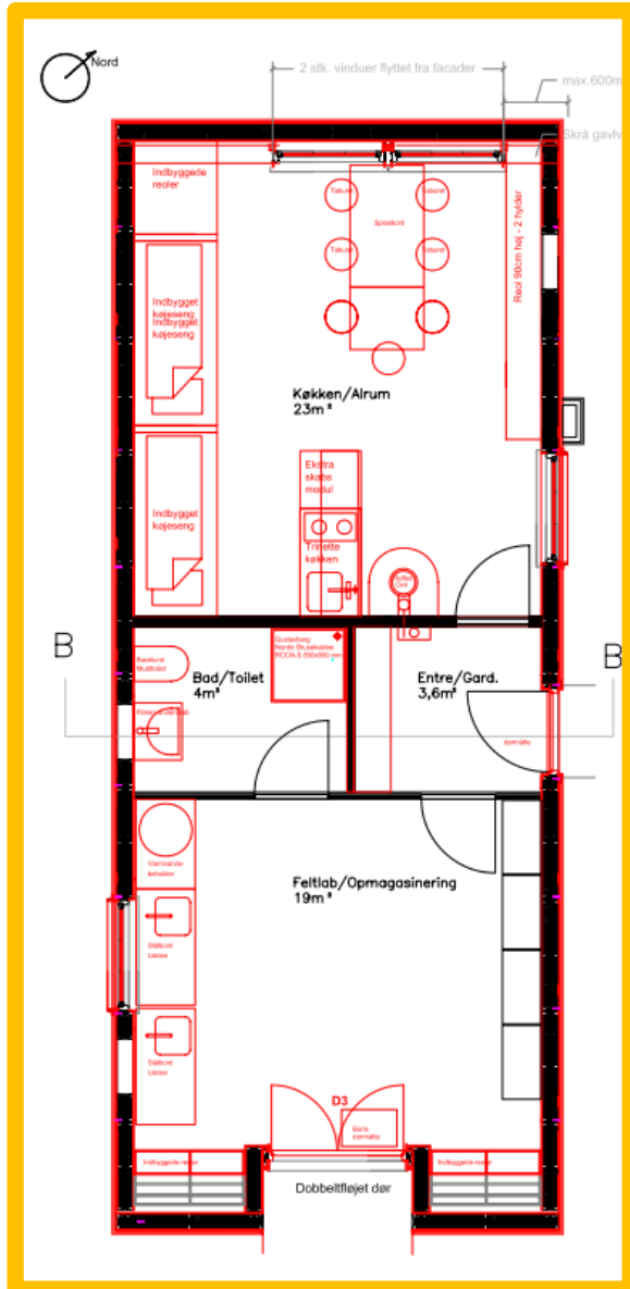
Plan af hytte, målestok 1:50
